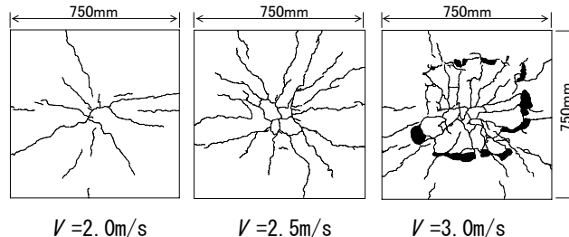
図-4 試験体下面の破壊状況（単一衝撃）
