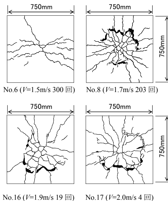
図-9 試験体下面のひび割れ発生状況 (繰返し衝撃)
