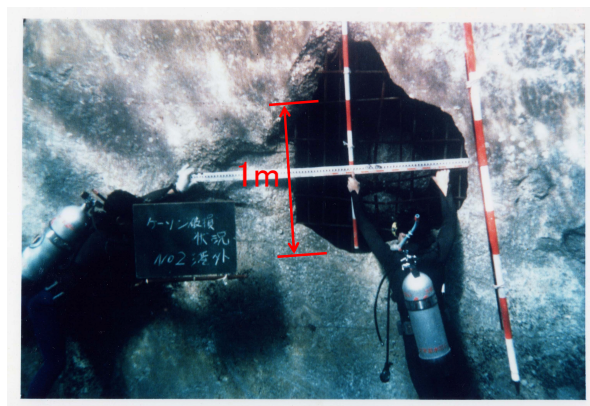
写真-1 貫通孔が生じた防波堤ケーソン壁の一例
