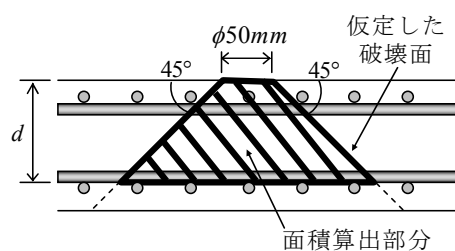
図-13 コーン破壊面の面積の考え方
