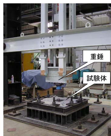
写真-2 衝撃載荷実験装置
