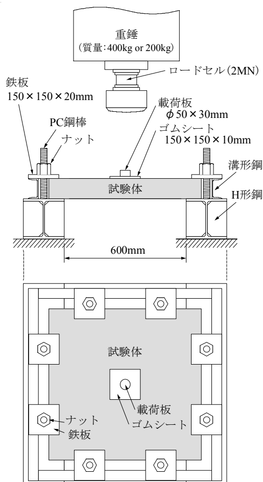
図-3 試験体設置部詳細
