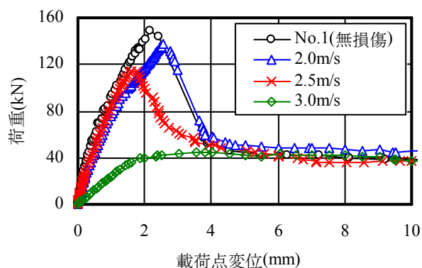
図-7 静的载荷実験による荷重と変位の関係
