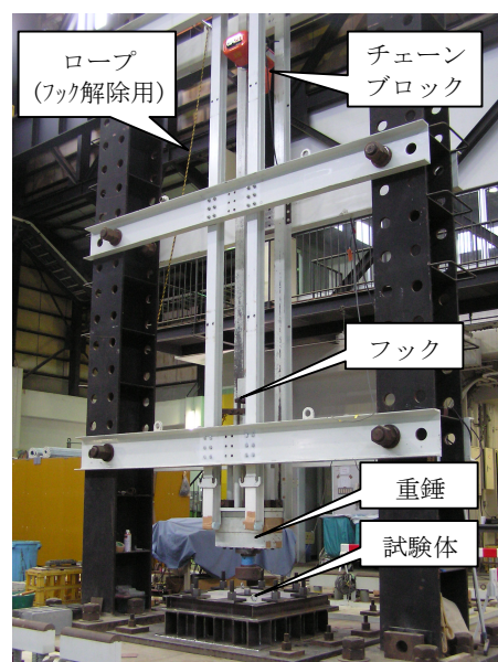
写真-2 衝撃試験装置全景
