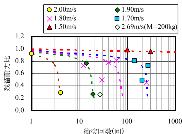
図-11 残留耐力比と衝突回数の関係
