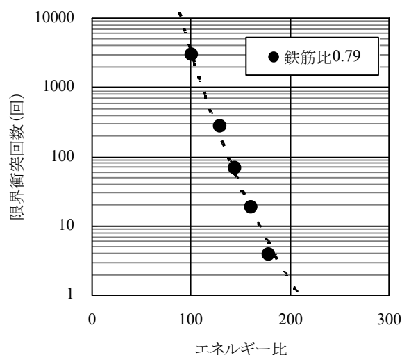
図-14 限界衝突回数とエネルギー比の関係
