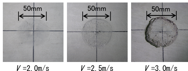
写真-4 衝突部の破壊状況（拡大写真）
