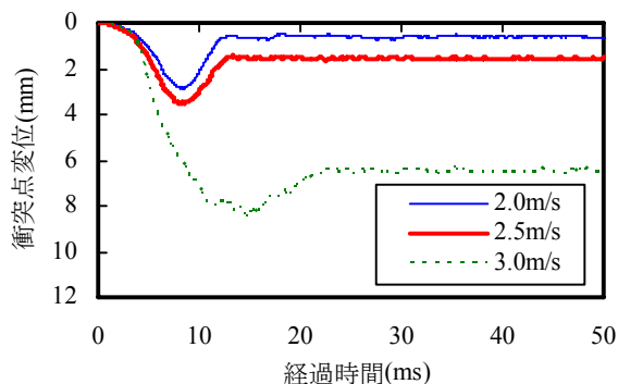
図-6 衝突点変位の時刻歴応答
