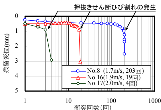
図-10 残留変位と衝突回数の関係
