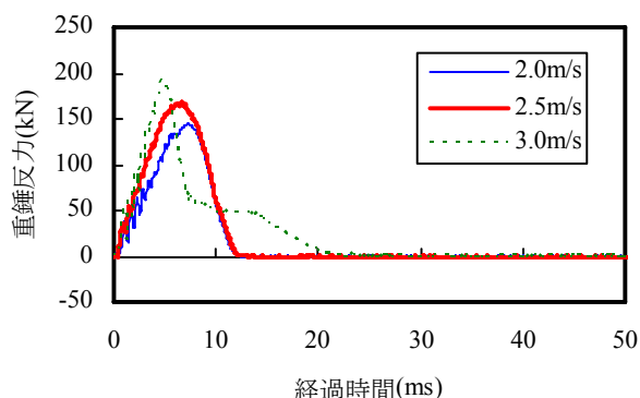
図-5 重錘反力の時刻歴応答
