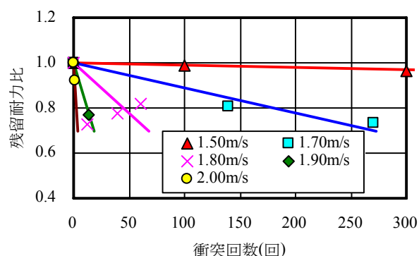
図-12 残留耐力比と衝突回数の関係
