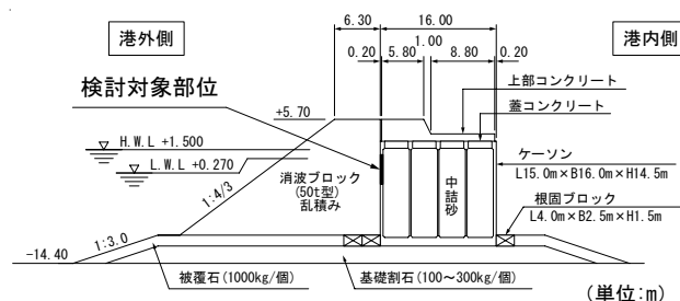
図-1 一般的な消波ブロック被覆堤の一例
