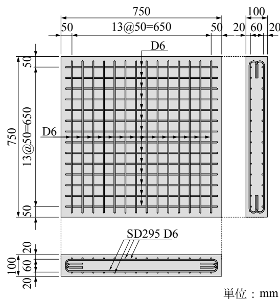
図-2 試験体形状および配筋
