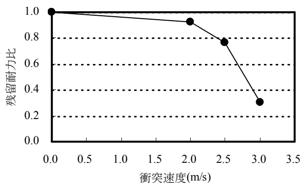
図-8 残留耐力比と衝突速度の関係
