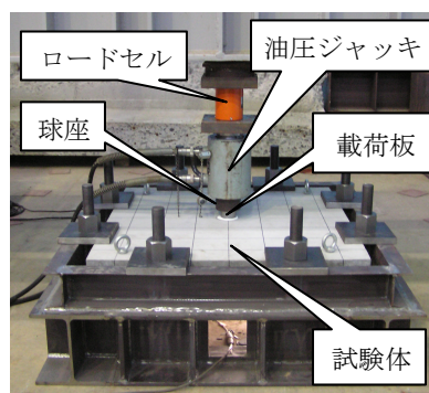
写真-3 静的載荷試験状況
