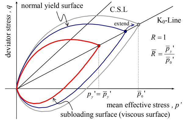
図-3 二次圧密による正規降伏曲面の移動
