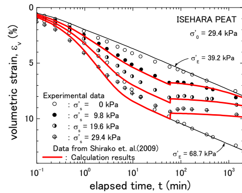
(b) 伊勢原泥炭の体積ひずみ経時変化
