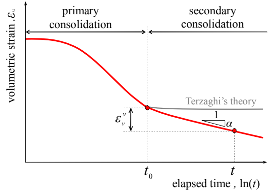
図-1 二次圧密による体積変化の模式図
