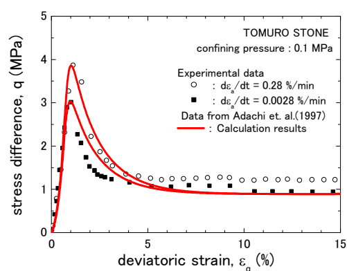
(b) 三軸排水せん断試験の応力～ひずみ関係
