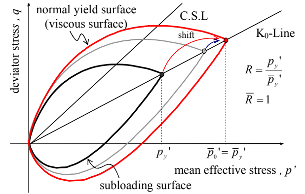
図-4 負荷・除荷を受けた場合の粘性曲面の移動
