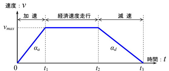
図-3 理想的な省燃費運転モデル 6)
