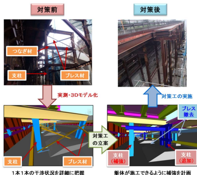
図-1 3次元モデルを活用した既設仮橋の干渉対策の立案
