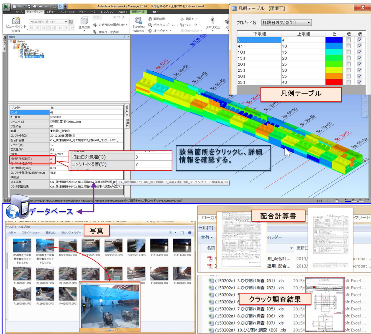
図-3 維持管理における CIM モデルの活用
