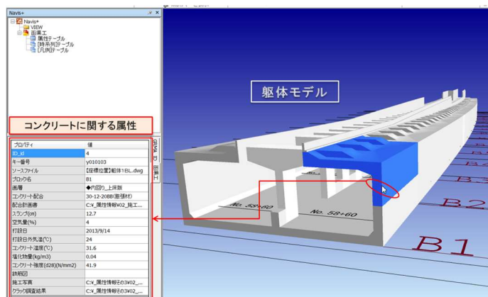
図-2 維持管理初期モデル
